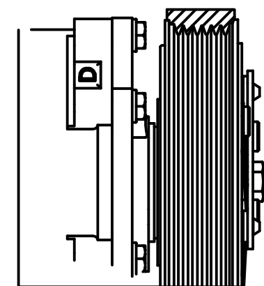
Схема расположения ремня на шкиве компрессора SD5H11
